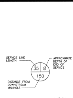
SEWER SERVICE SYMBOL N.T.S.
