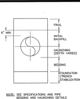
TRENCH TERMINOLOGY N.T.S.
